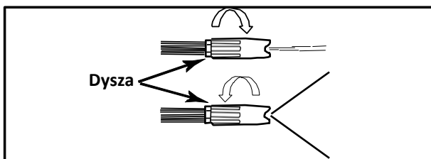
Rysunek 2 - Regulacja dyszy w celu uzyskania wzoru wachlarza (nie dotyczy niektórych dysz)
