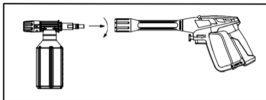
Rysunek 8 - Mocowanie aplikatora do pistoletu
