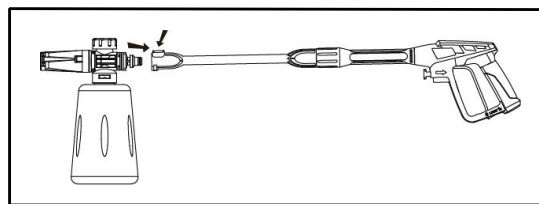
Figure 8 - Fixer l'applicateur au pistolet
